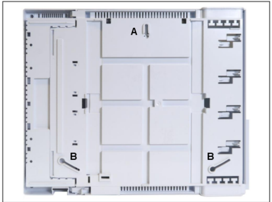
Abbildung 1: OpenScape Business X1 – Befestigungslöcher in der Gehäuserückwand
