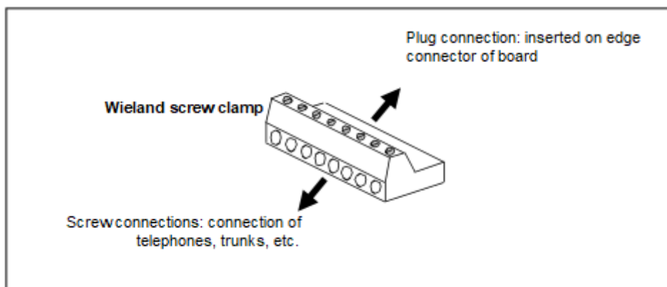
Abbildung 3: Wieland-Schraubklemmen
